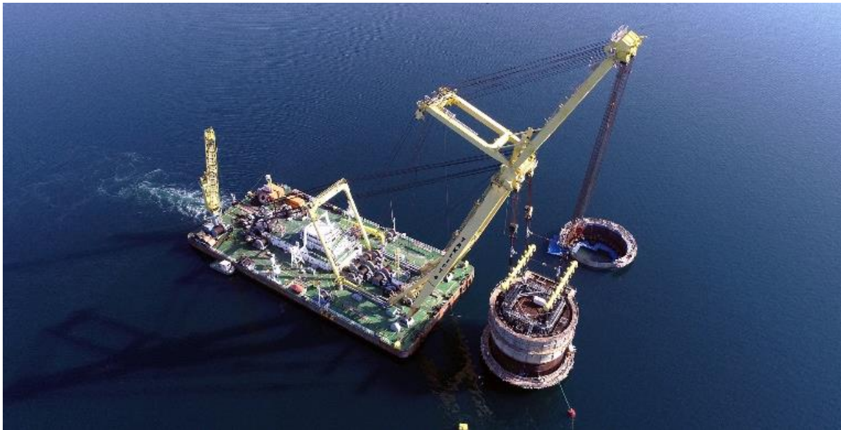
Hijswerkzaamheden voor de Çanakkale 1915 Brug door de drijvende bok Taklift 4 van Boskalis in 2019
